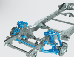
HỆ THỐNG TREO TRƯỚC TAY ĐÒN KÉP
