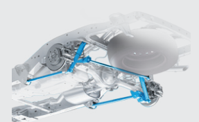
HỆ THỐNG TREO SAU ĐA LIÊN KẾT
